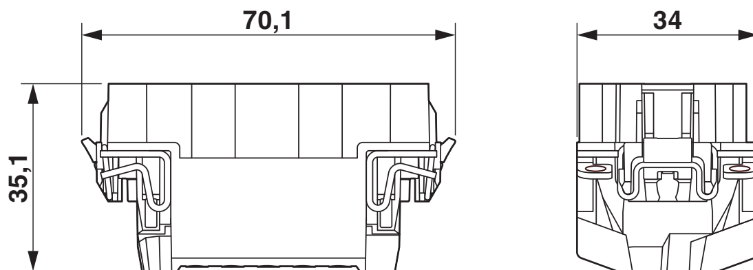
Dessin coté
