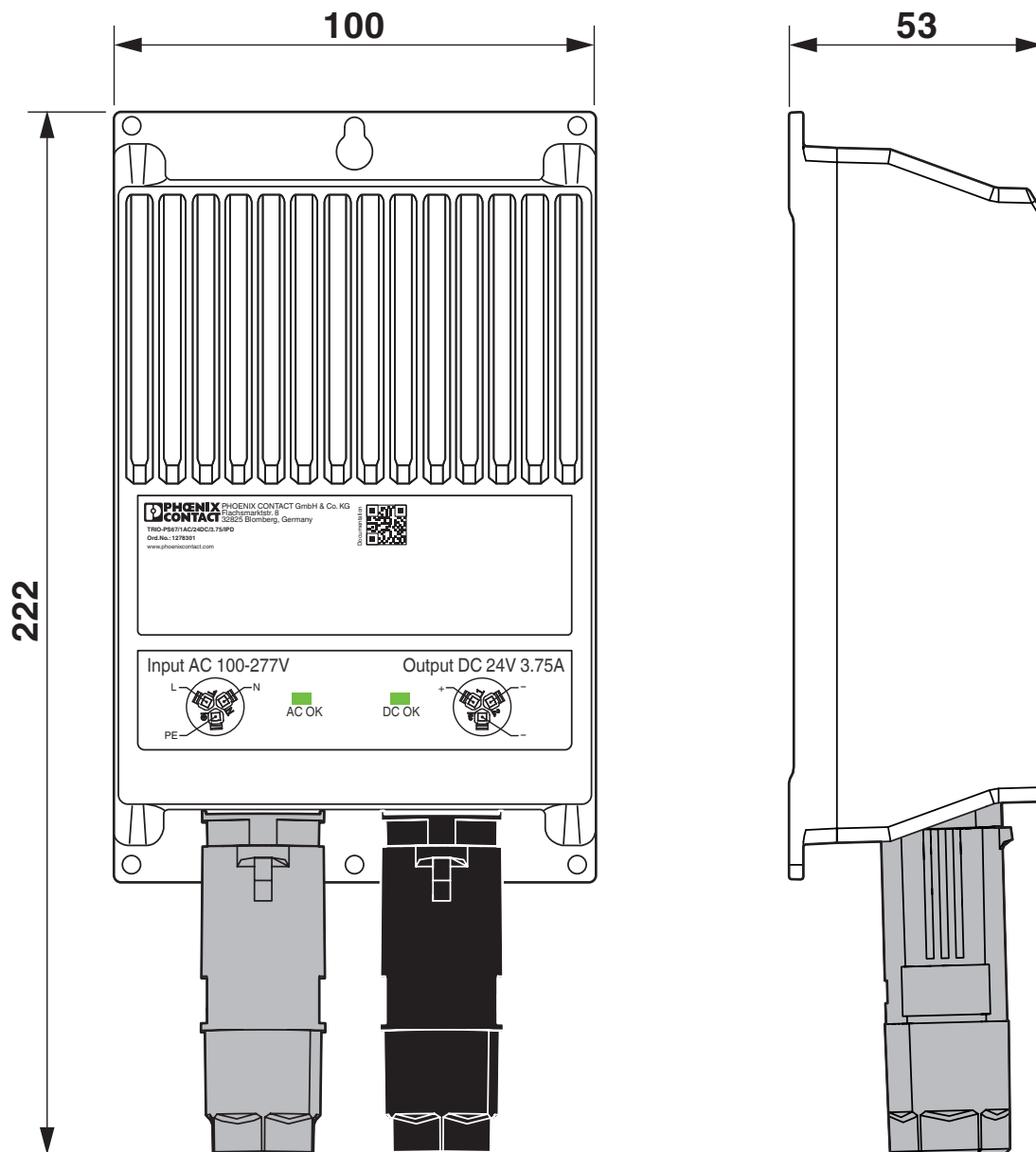
Dessin coté
