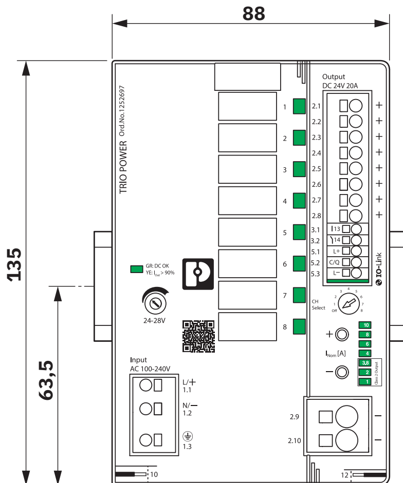
Dessin coté
