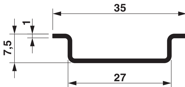
Dessin coté
