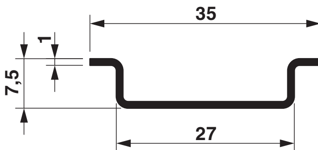
Dessin coté
