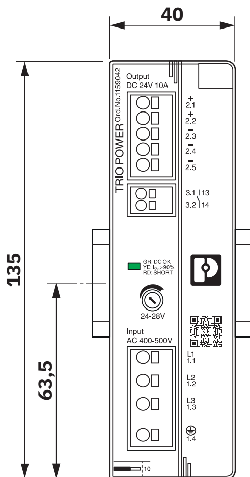
Dessin coté
