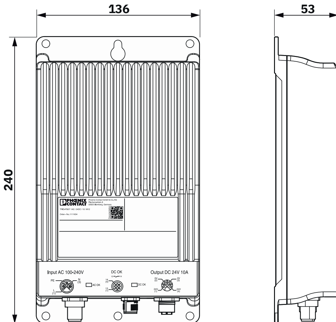
Dessin coté
