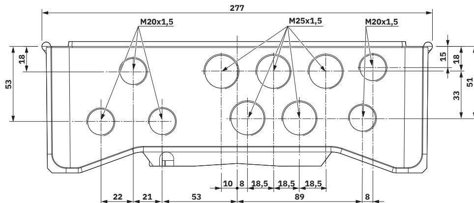
Dimensions de la face inférieure
