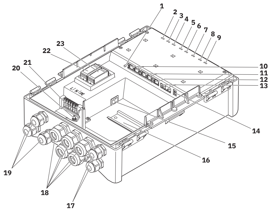
Dessin schématique
