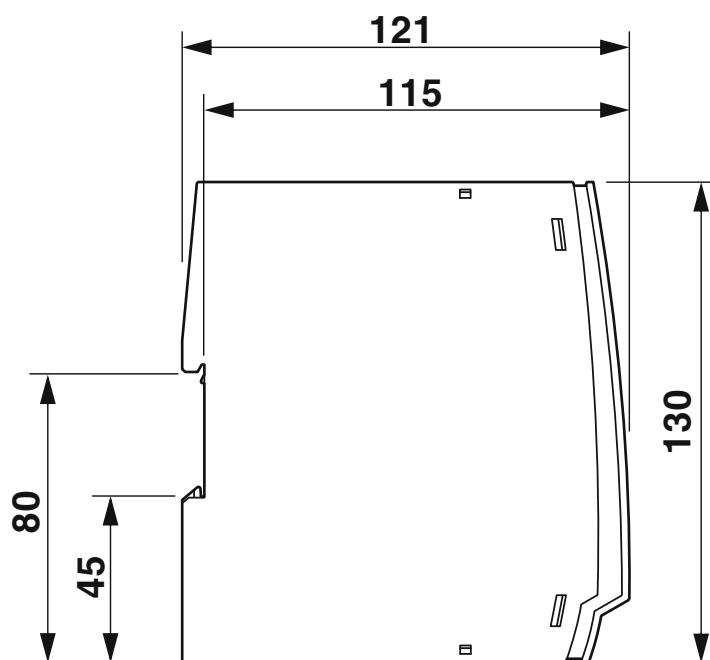
Dessin coté
