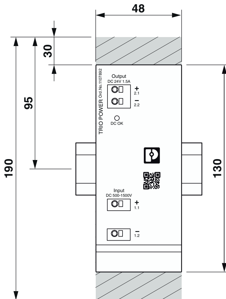
Dessin coté
