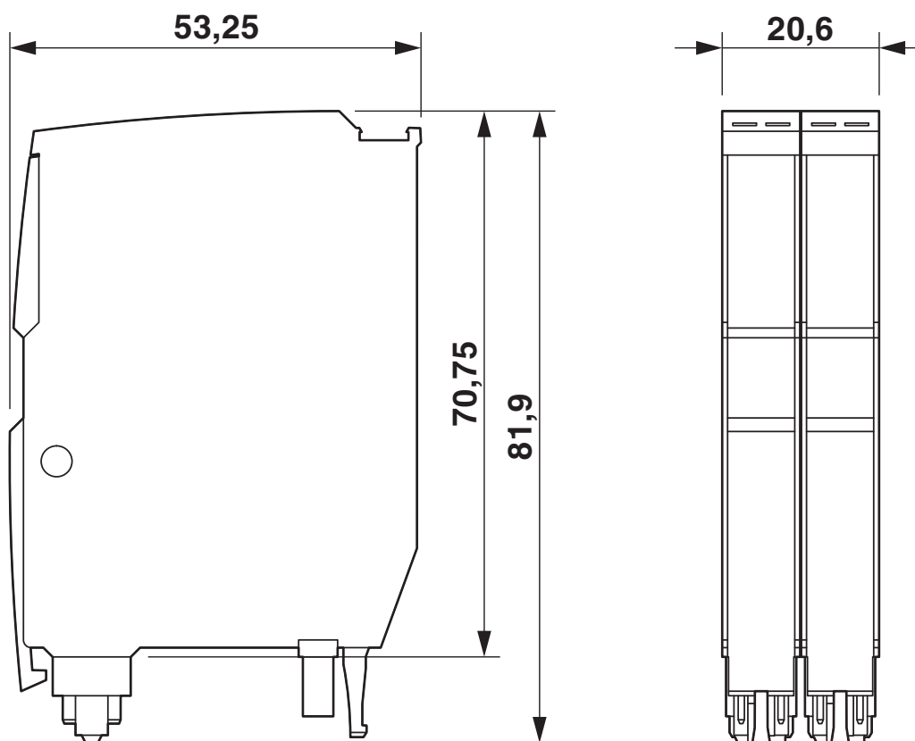
Dessin coté
