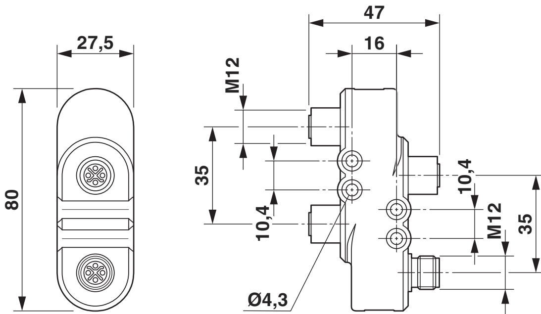
Dessin coté
