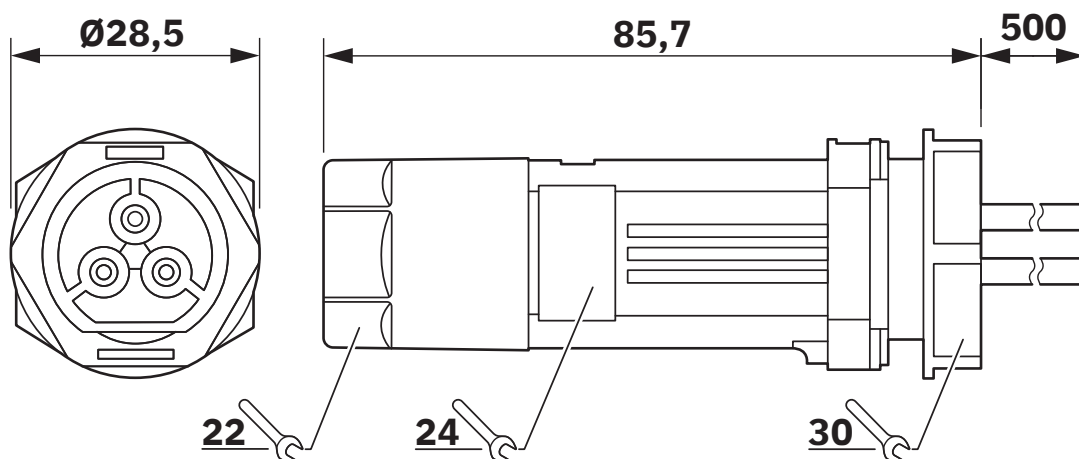
Dessin coté
