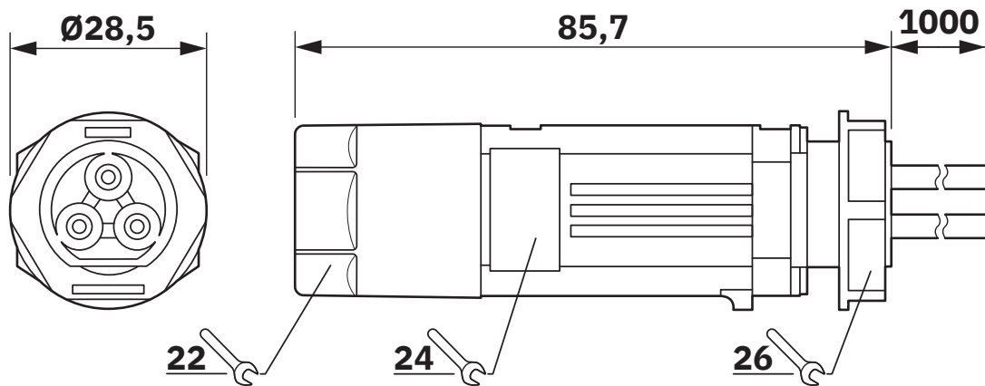
Dessin coté
