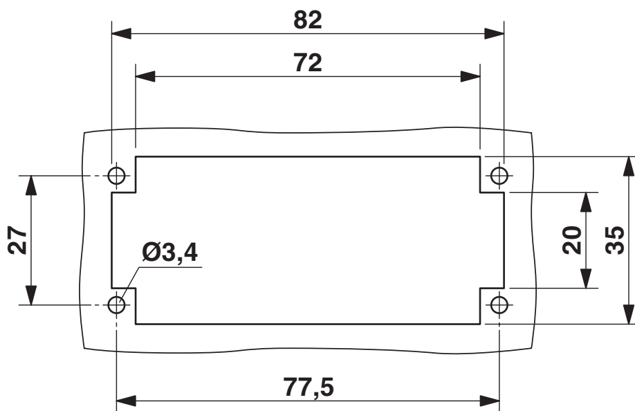
Dessin coté
