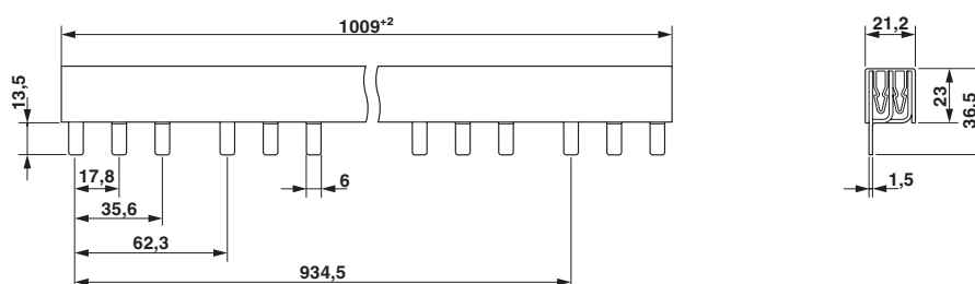
Dessin coté
