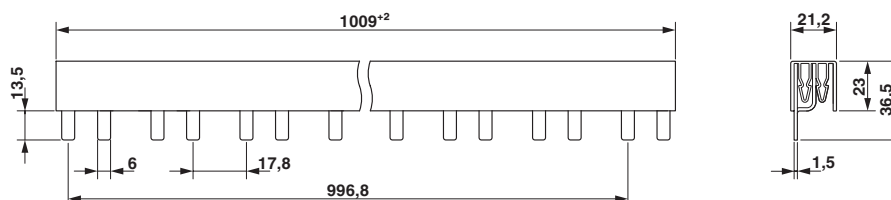
Dessin coté
