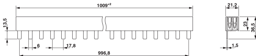
Dessin coté
