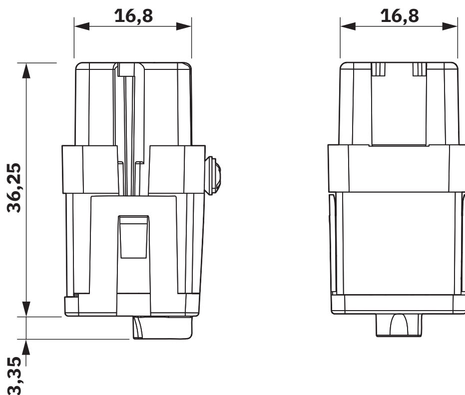
Dessin coté
