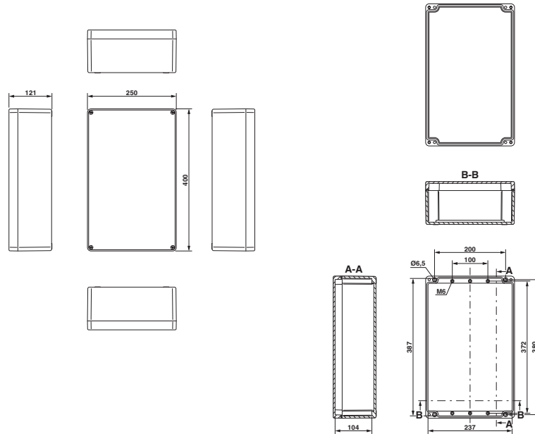
Dessin coté
