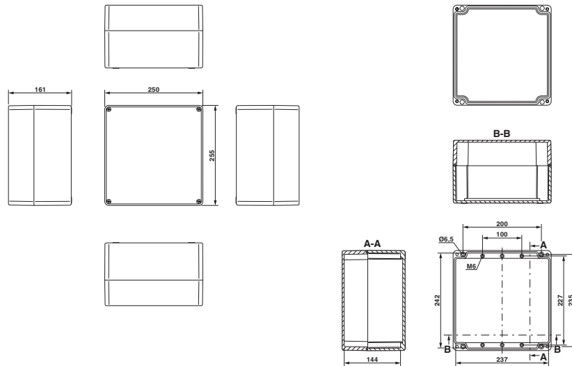
Dessin coté
