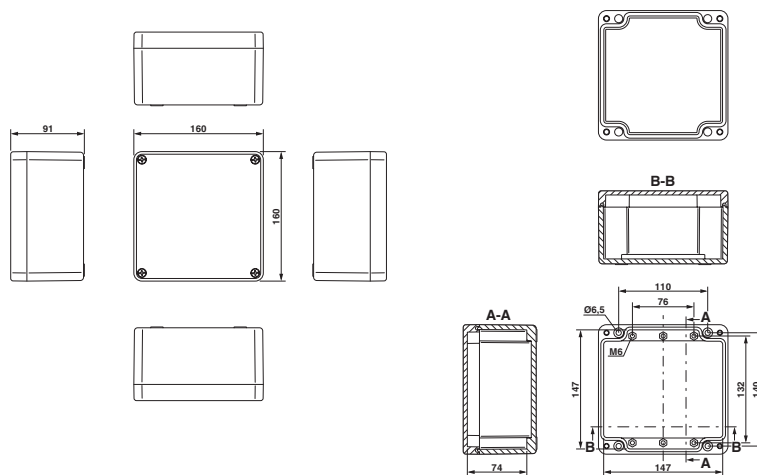
Dessin coté
