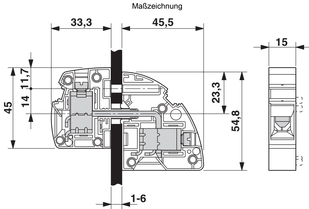
Maßzeichnung
