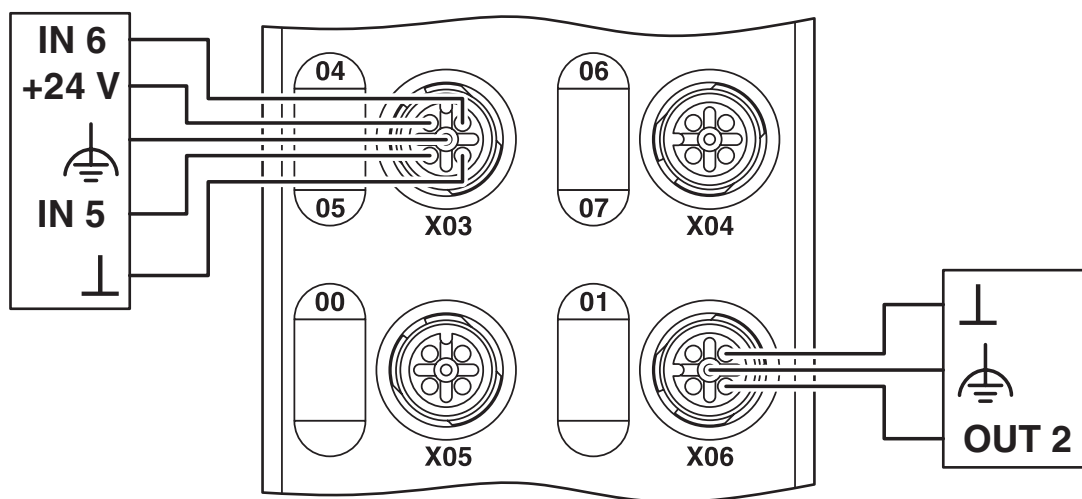
Anschlusszeichnung
