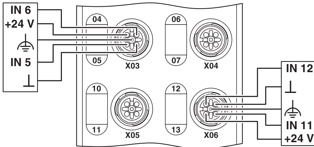
Anschlusszeichnung
