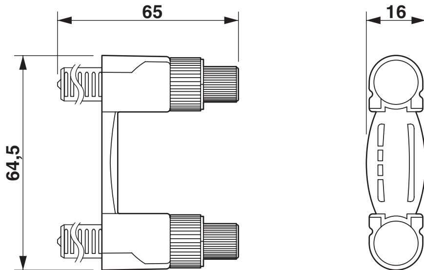
Maßzeichnung
