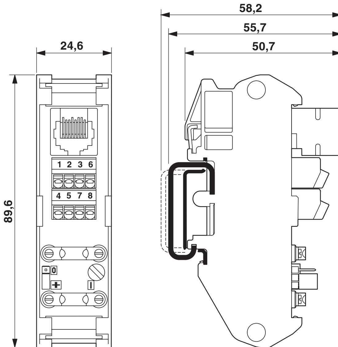
Maßzeichnung
