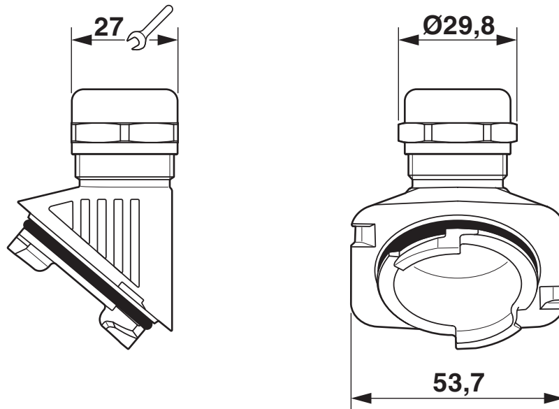
Maßzeichnung
