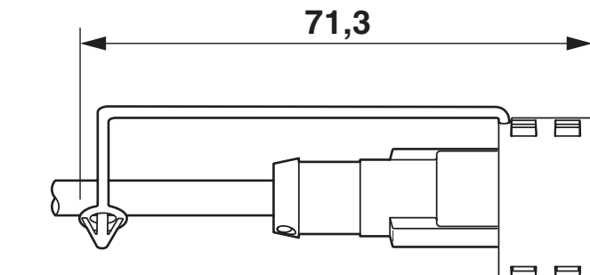
Maßzeichnung
