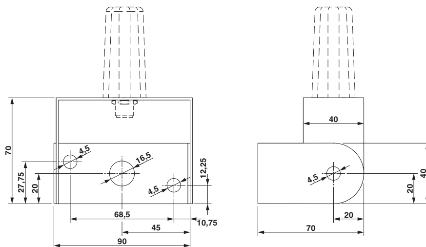
Maßzeichnung
