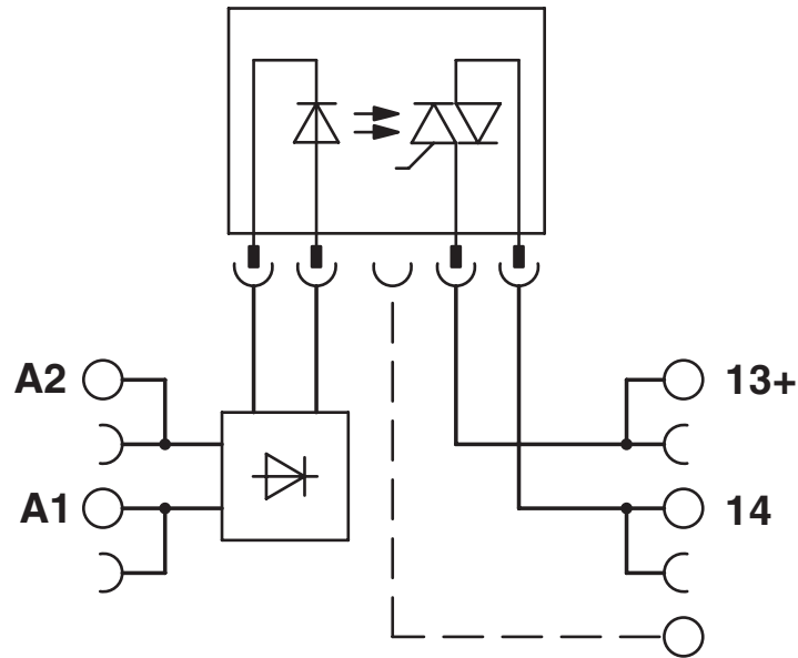
Schaltplan
