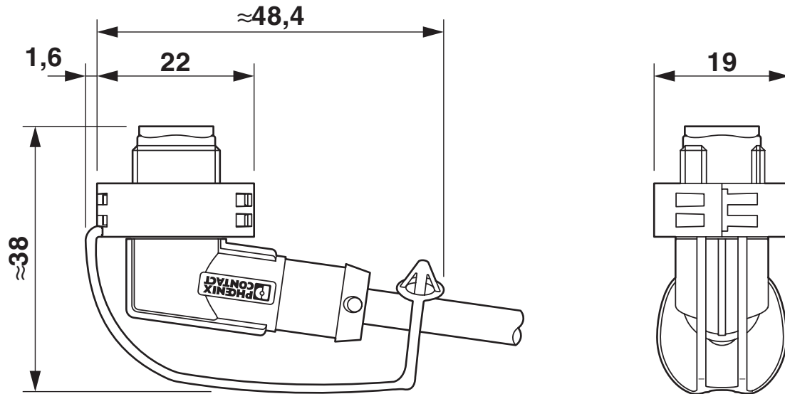
Mit EXCLIP montierter Stecker
