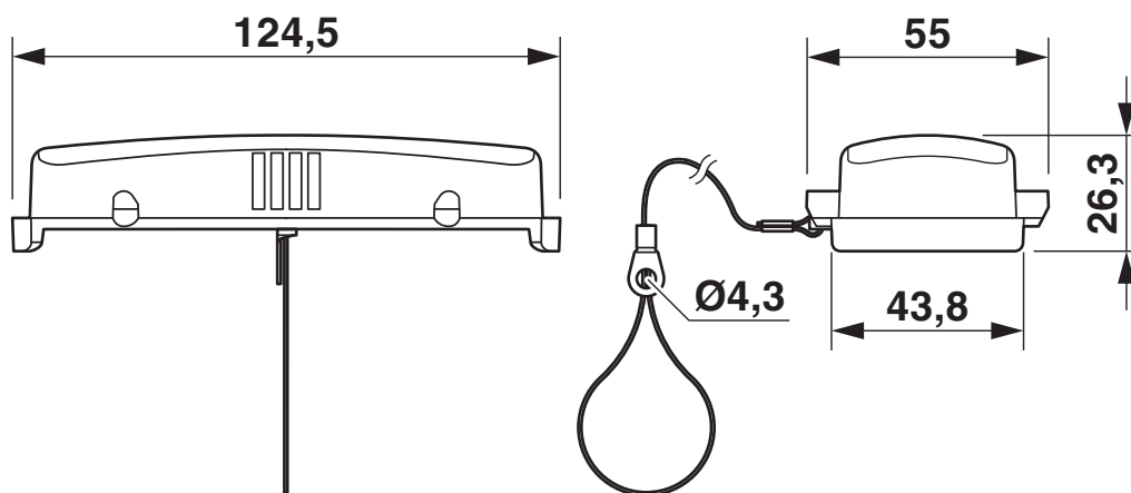
Maßzeichnung
