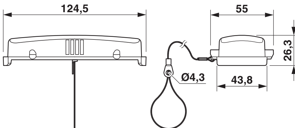
Maßzeichnung
