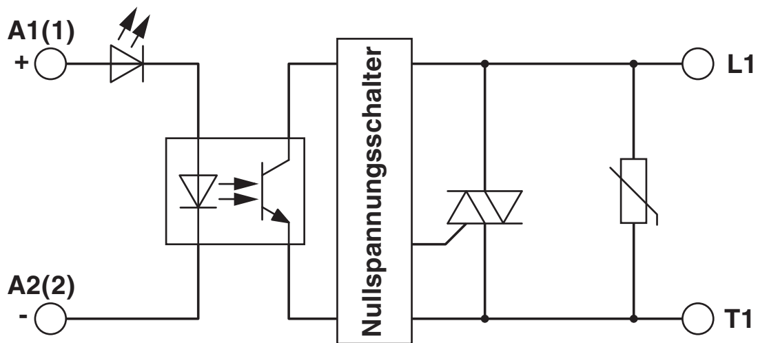
Blockschaltbild
