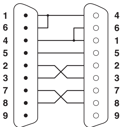
Diagrama de circuitos
