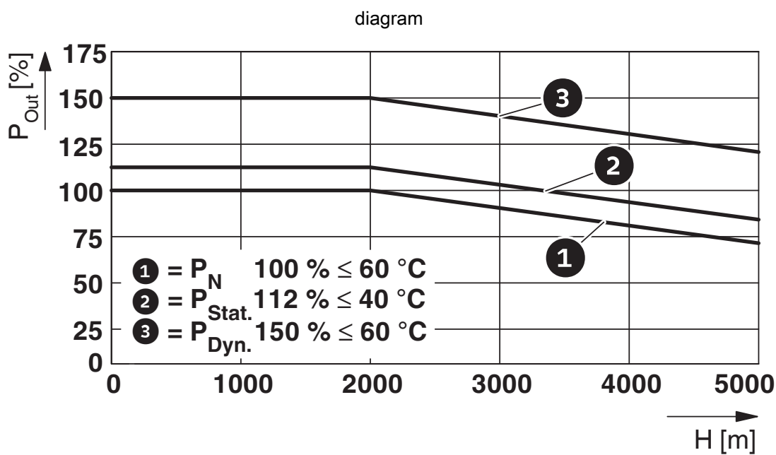
Hoogte-afhankelijke derating
