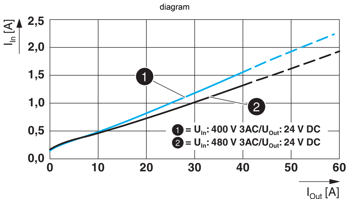
Ingangsstrom/uitgangsstrom
