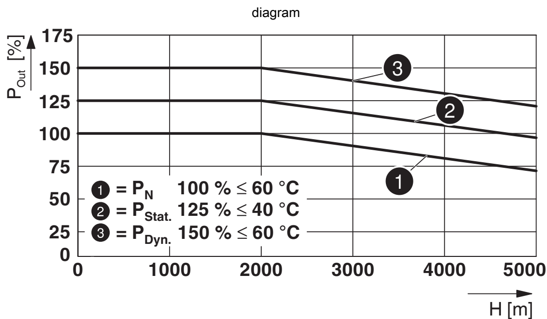
Hoogte-afhankelijke derating
