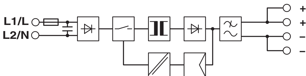
blokschema
