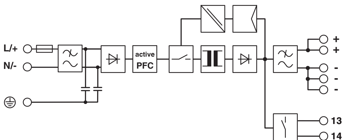
blokschema
