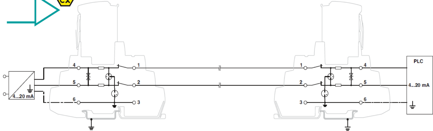
TTC-6P-1X2-M-EX-24DC-UT-I
