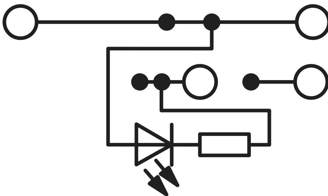
Kopplingsschema
