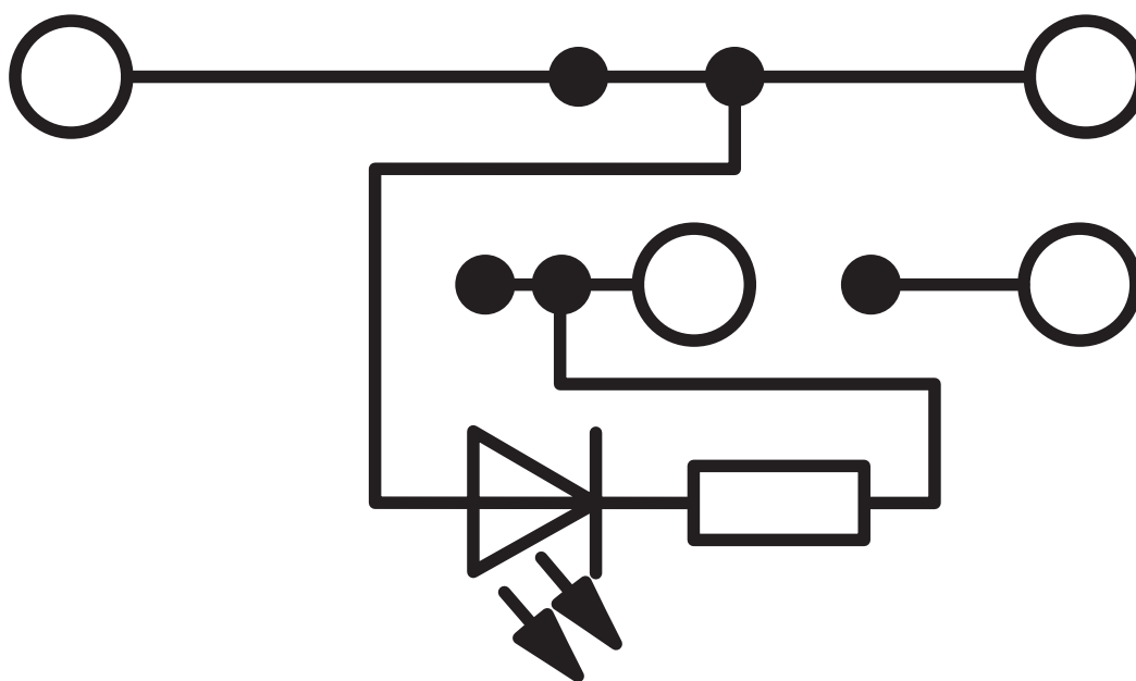
Kopplingsschema
