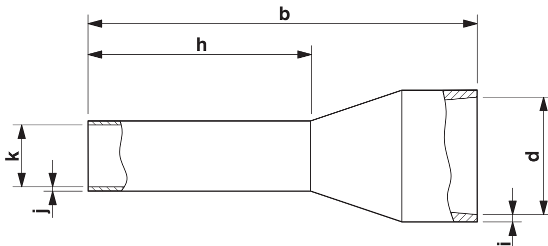
Måttskiss
