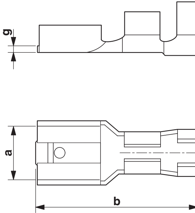
Måttskiss
