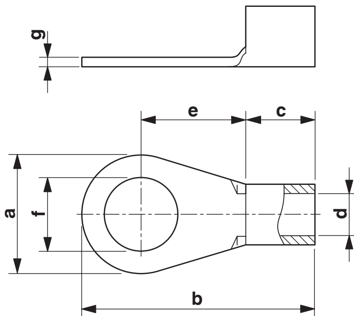
Måttskiss
