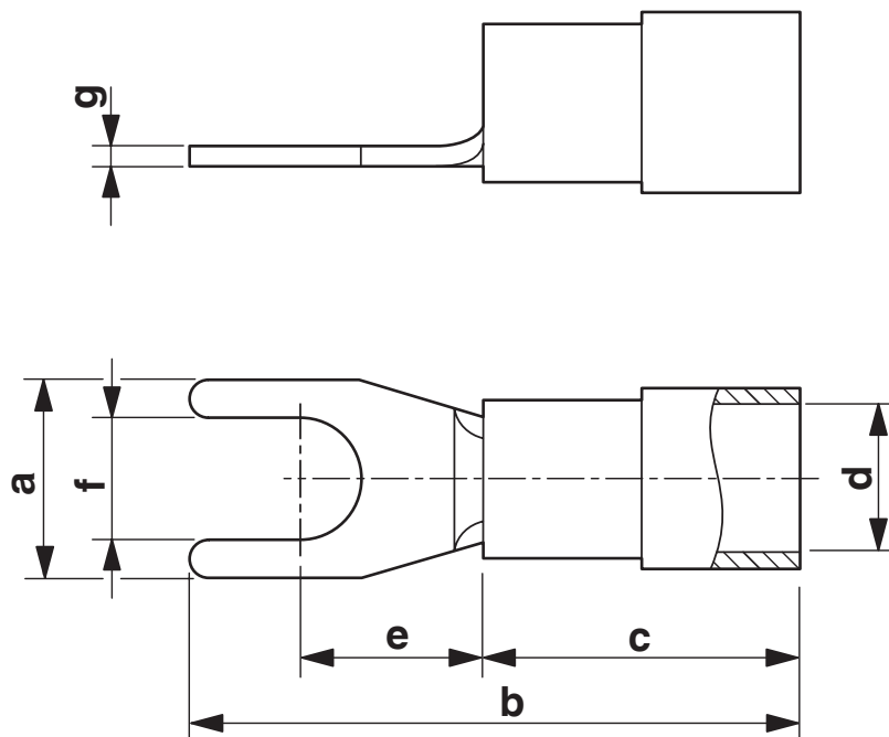
Måttskiss
