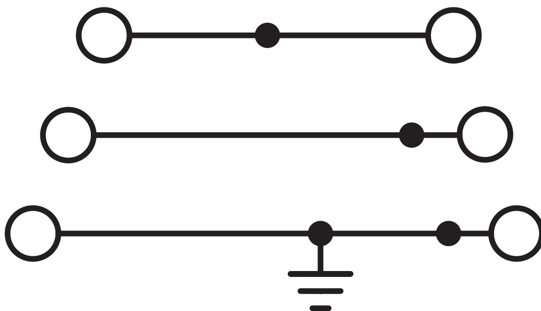
Kopplingsschema
