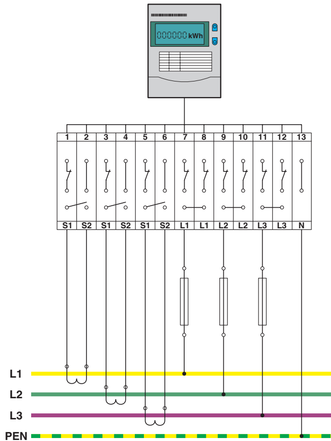
Kopplingsschema
