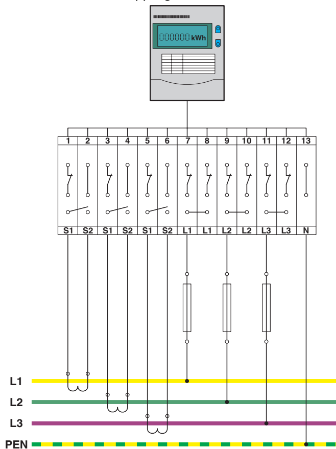
Kopplingsschema
