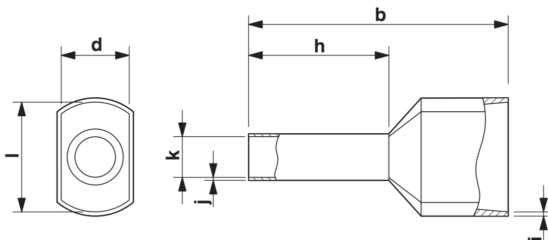
Måttskiss
