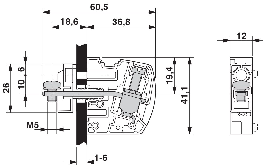
Måttskiss
